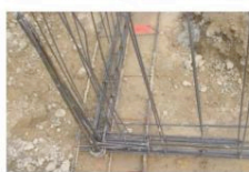
Noeud de chaînage - Continuité mécanique
