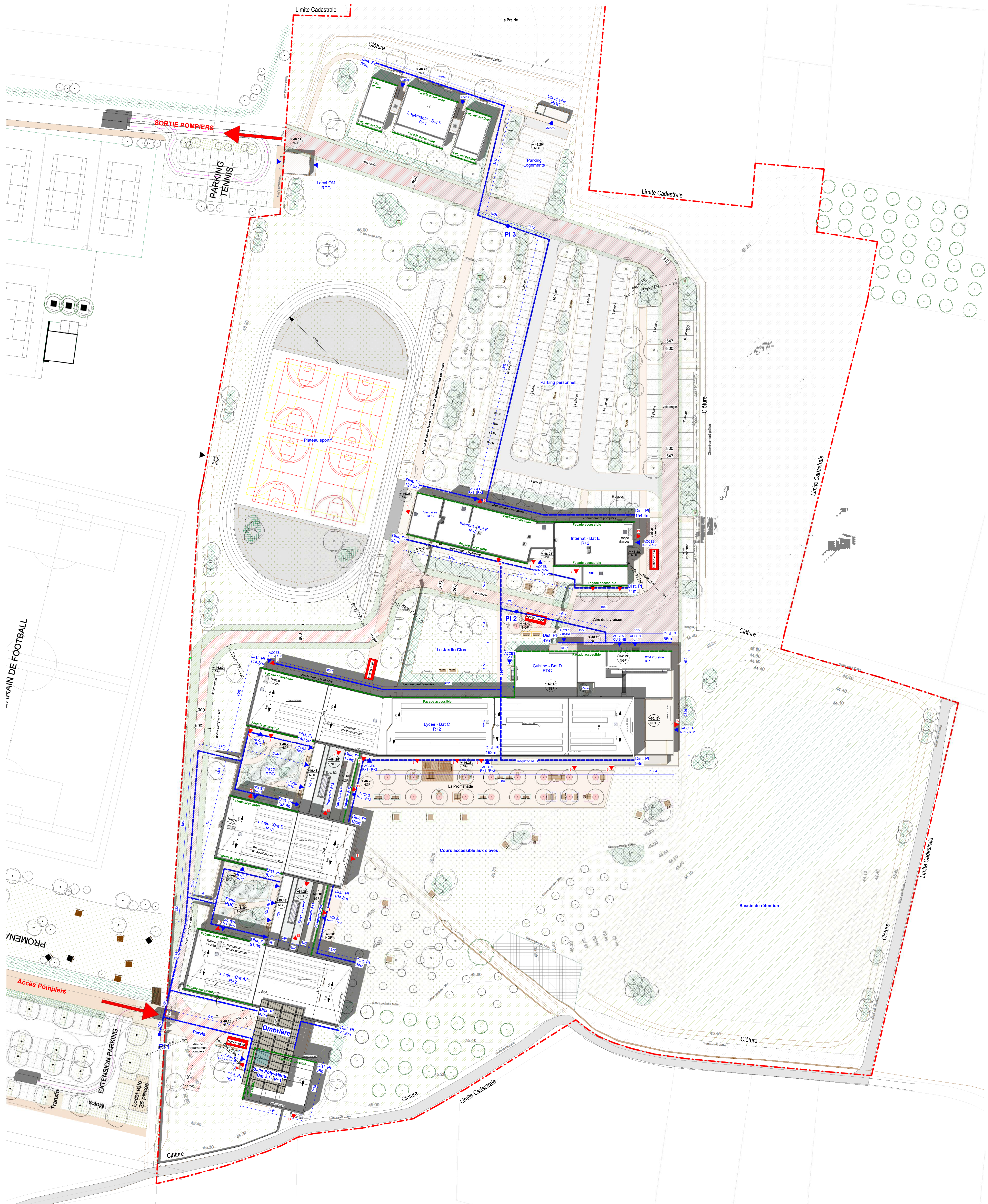
Plan de Masse 1:500
